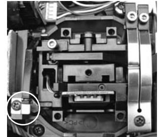
Ausgehobene Rückstellfeder für Drossel links (Mode 2 + 4)
