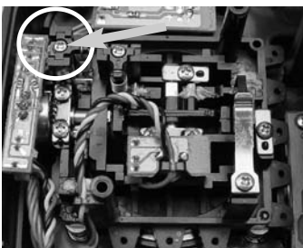
Pos. 6 Feder an der linken vertikalen Neutralisierungswippe aushängen. Wippe vorsichtig entfernen.
